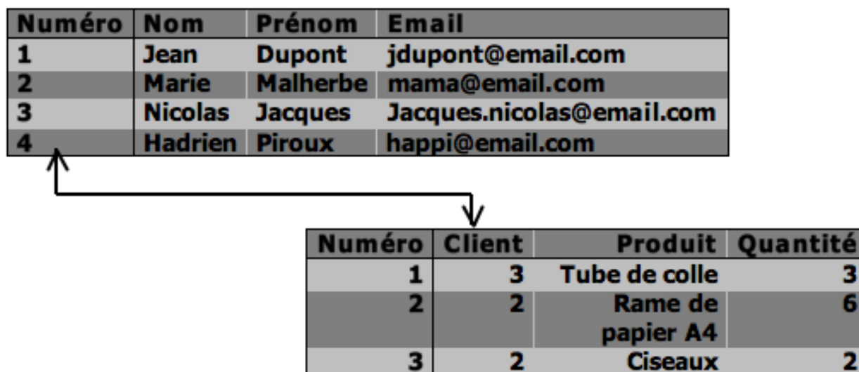
FIGURE II.2.1. – Référence d'une table à une autre
