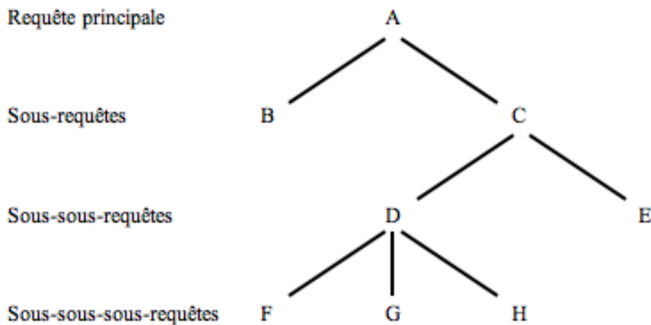
FIGURE II.4.1. – Sous-requêtes corrélées
