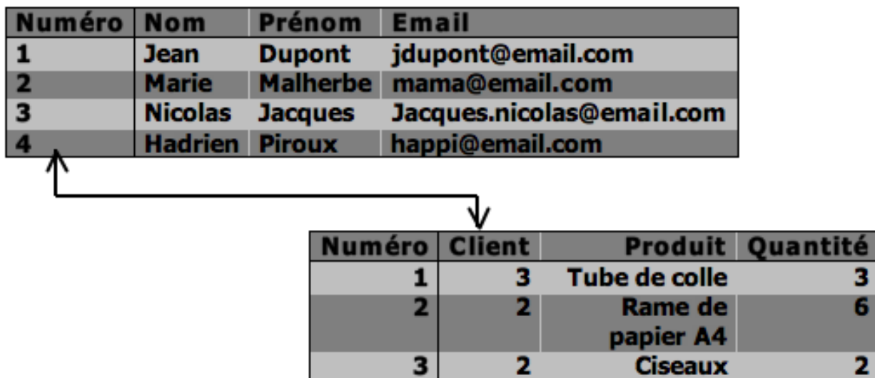
FIGURE I.1.1. – Schéma bdd relationnelle
