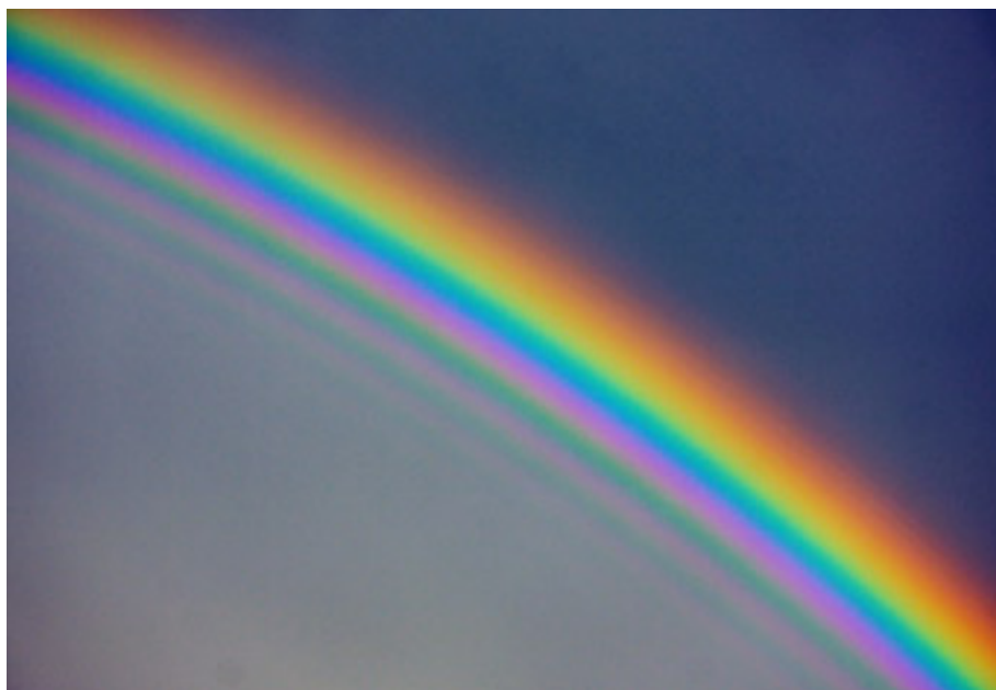
FIGURE 4. – Détail des franges surnuméraires d'un arc-en-ciel. © Jean-Marc Leclaire/astroturf.fr
