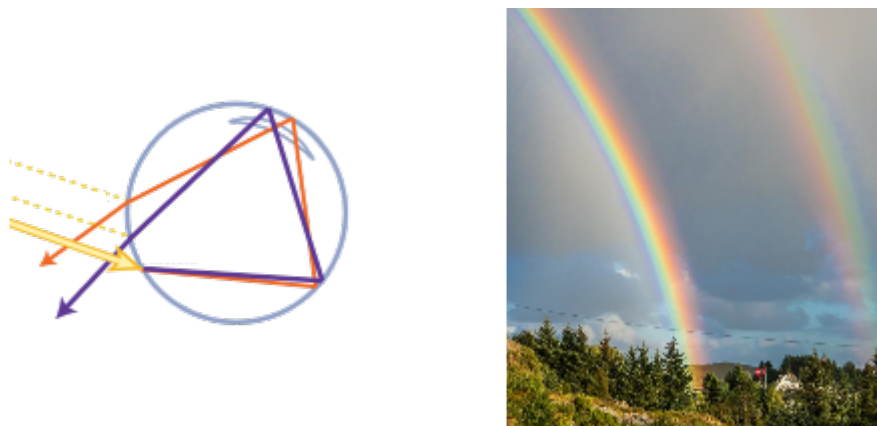
FIGURE 3. – À gauche, schéma d'une double réflexion dans une goutte. À droite, un arc-en-ciel double. © sciencecalculators.org et © Mikhail Varentsov
